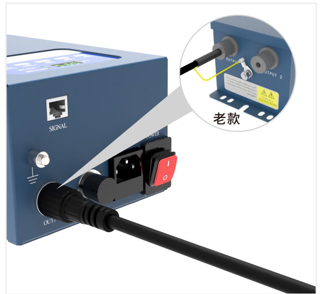
全新高压输出端口，与静电棒无外接地线设计的高压插头连接使用，安全性能更高
